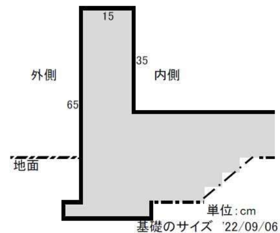
基礎断面図
